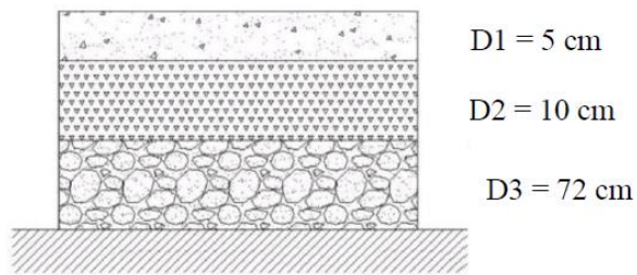
Gambar 6: Susunan Lapisan Perkerasan Lentur
